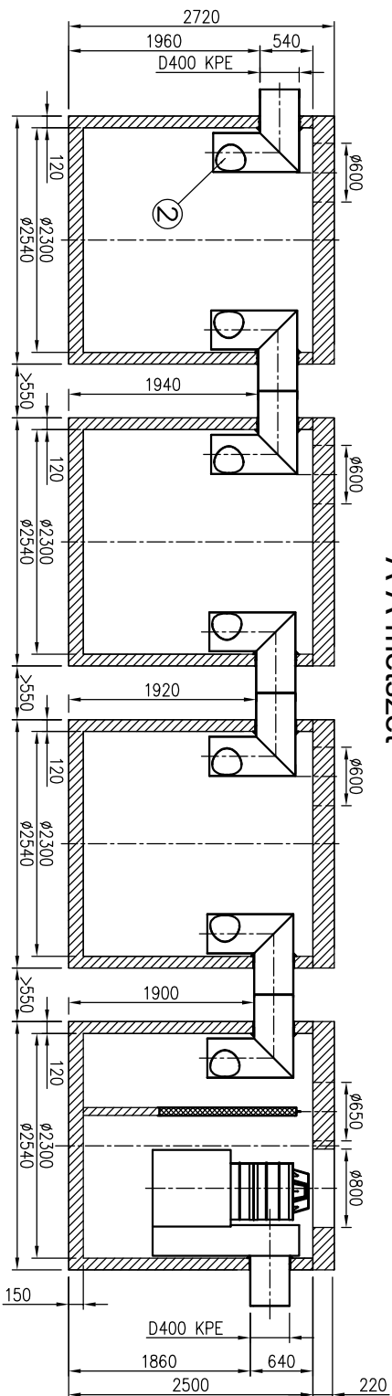
Felülnézet
