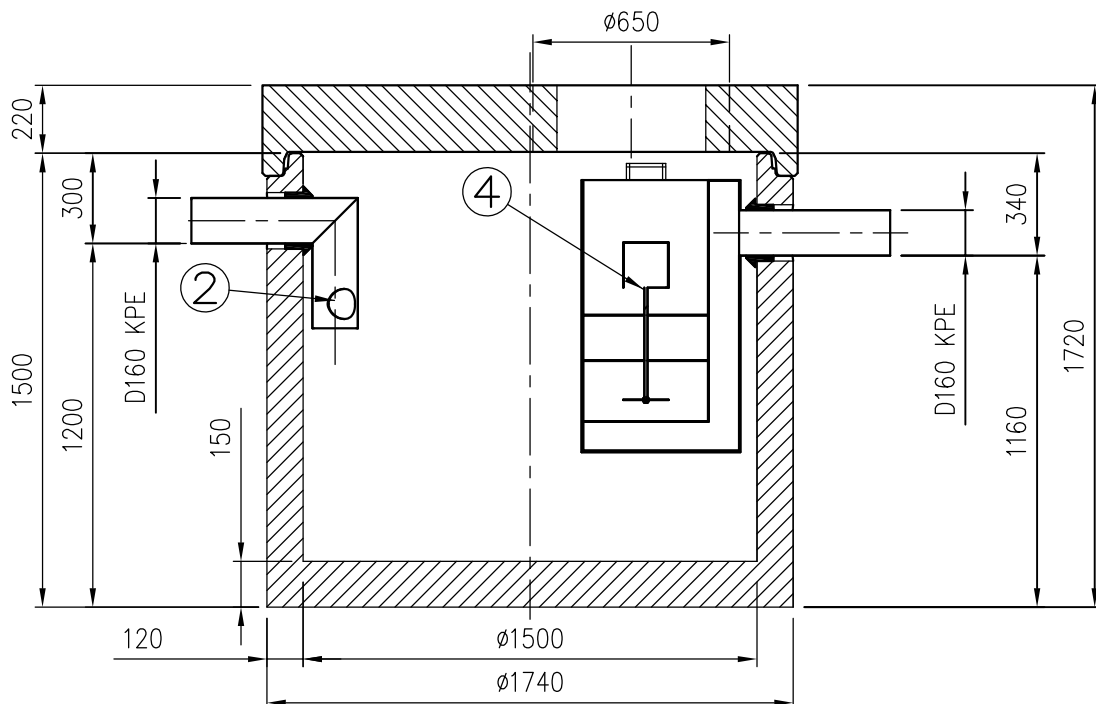
A-A metszet
